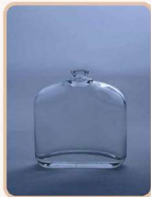
HY-X0270 H: 98mm W: 240g S: 94*34mm V: 120ml
